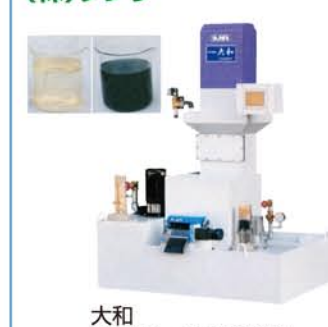
大和 超精密クーラント濾過装置
