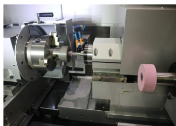
2 軸単軸駆動方式
