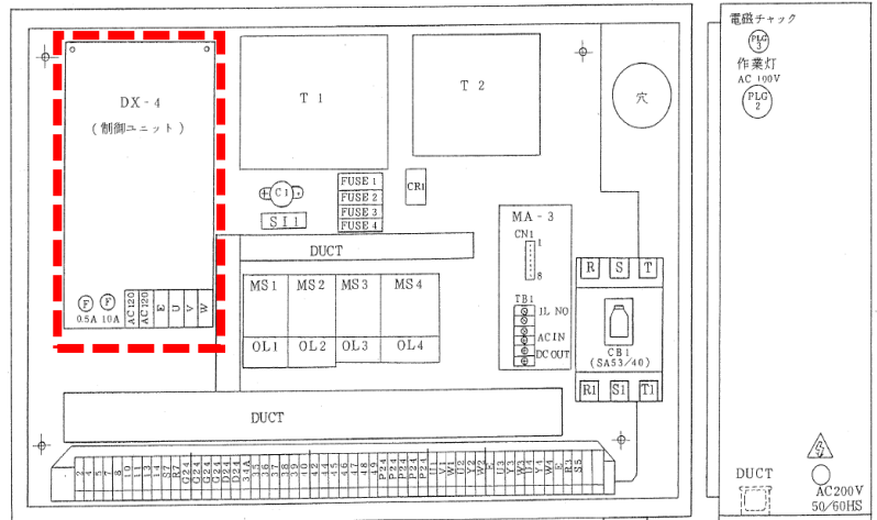
旧・電装BOX内部
